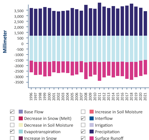
Figura 7. Modelo hidrológico de dos tanques WEAP cuenca alta del río Caquetá.
