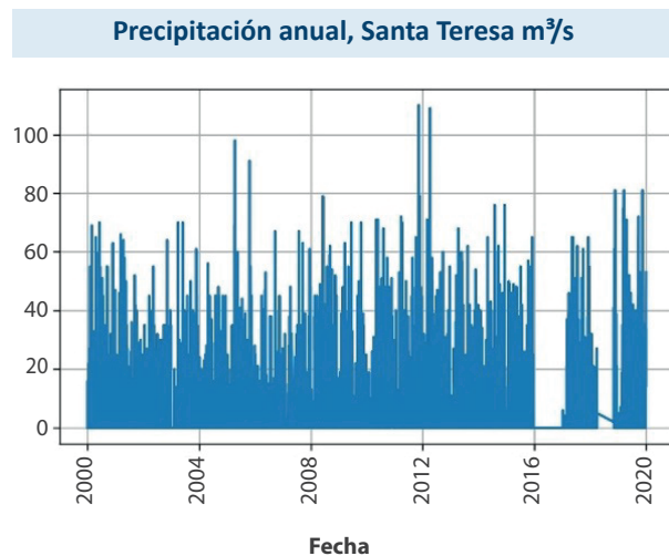
Figura 7. Precipitación anual en la Estación Santa Teresa en el periodo 2000 - 2020. Fuente: Elaboración Propia.
