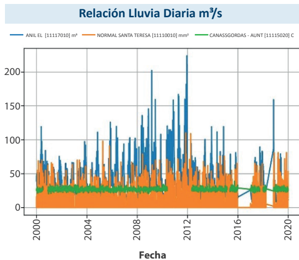
Figura 11. Relación de la precipitación diaria, caudal y temperatura. Fuente: Elaboración Propia.
