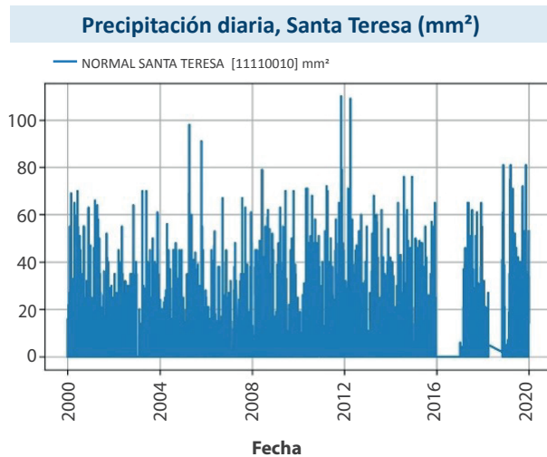
Figura 6. Precipitación diaria en la Estación Santa Teresa en el periodo 2000 - 2020. Fuente: Elaboración Propia.
