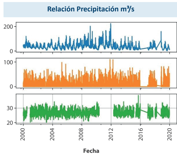
Figura 10. Relación de la precipitación, caudal y temperatura. Fuente: Elaboración Propia.
