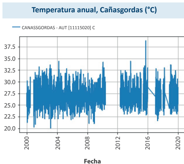
Figura 9. Temperatura media anual en la Estación Cañasgordas. Fuente: Elaboración Propia.
