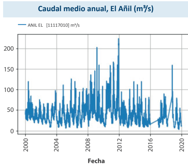
Figura 5. Caudal medio anual en el periodo 2000 - 2020. Fuente: Elaboración Propia.
