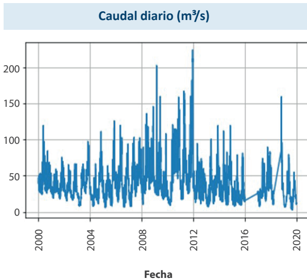
Figura 4. Caudal medio diario en el periodo 2000 - 2020. Fuente: Elaboración Propia.
